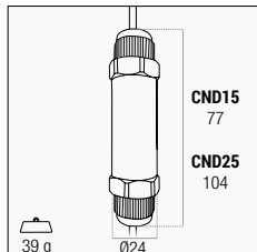
LINEARE 2 VIE / LINEAR 2 WAY
