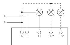
Schema di collegamento interruttore Switch connection diagram
