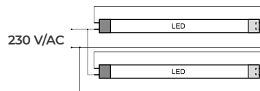
Cablaggio doppio tubo interno. Internal double tube wiring.
